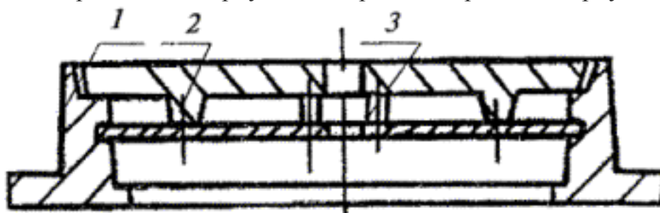
Рисунок А.1 - Люк общего назначения
